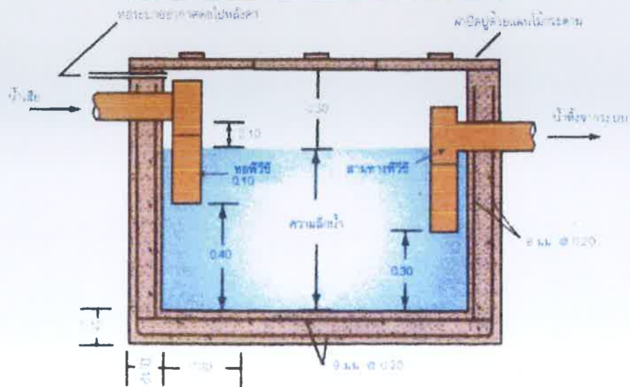
บ่อตกไข่แบบสร้างในที่สำหรับอาคารขนาดใหญ่
