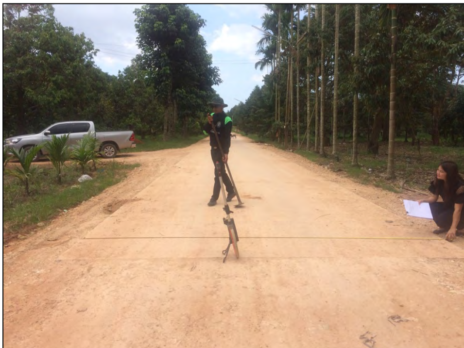
ภาพถ่ายโครงการก่อสร้างถนนคอนกรีตเสริมเหล็ก ซอยบ่อทราย 1 หมู่ที่ 2
